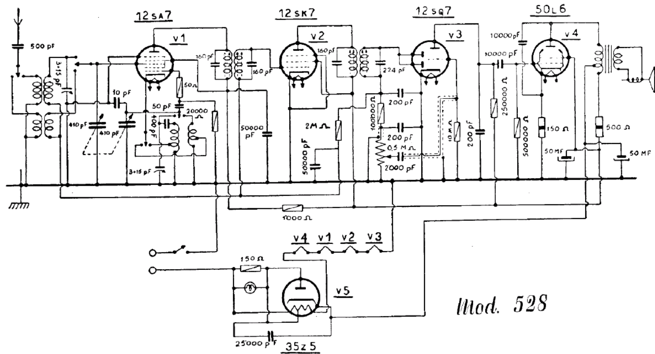
RADIO SUPERLA - Mod. 528 - Ad alimentazione diretta. Gamma onde medie (da 200 a 590 m) e corte (da 16 a 54 m). Media frequenza: 468,5 kc. Altoparlante a magnete permanente. Potenza d'uscita: 2 W. Un capo della rete-luce è collegato al telaio.
